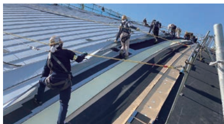
15人以上を配置して不整形の屋根材を葺く
