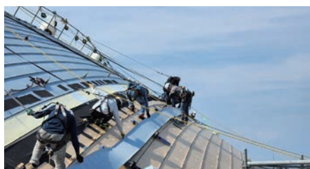
端部に近くなると勾配がきつくなり、安全管理に細心の注意をはらう
