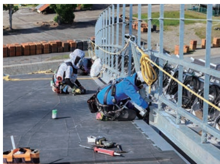
軒樋の取り付け。直線のない軒は事前に何度も実測を重ねても納めが難しい
