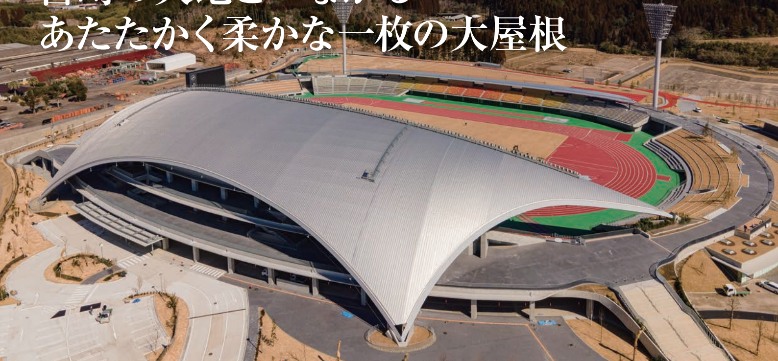
上空から。KUROKIRI STADIUM 楕円や球体で構成された「角」がほばない競技場。柔らかく人を誘うような動線、スタジアムの臨場感を考えた計画
