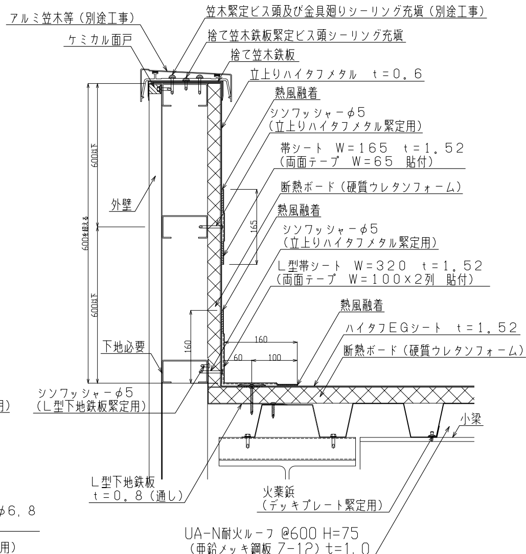
＜立上り高さ600mmを超える場合＞
